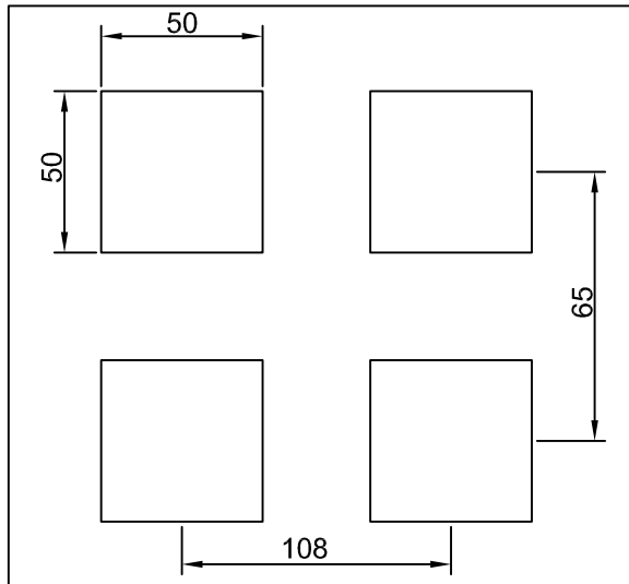
Fundamentplan Octo
