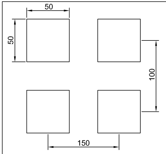
Fundamentplan Solido
